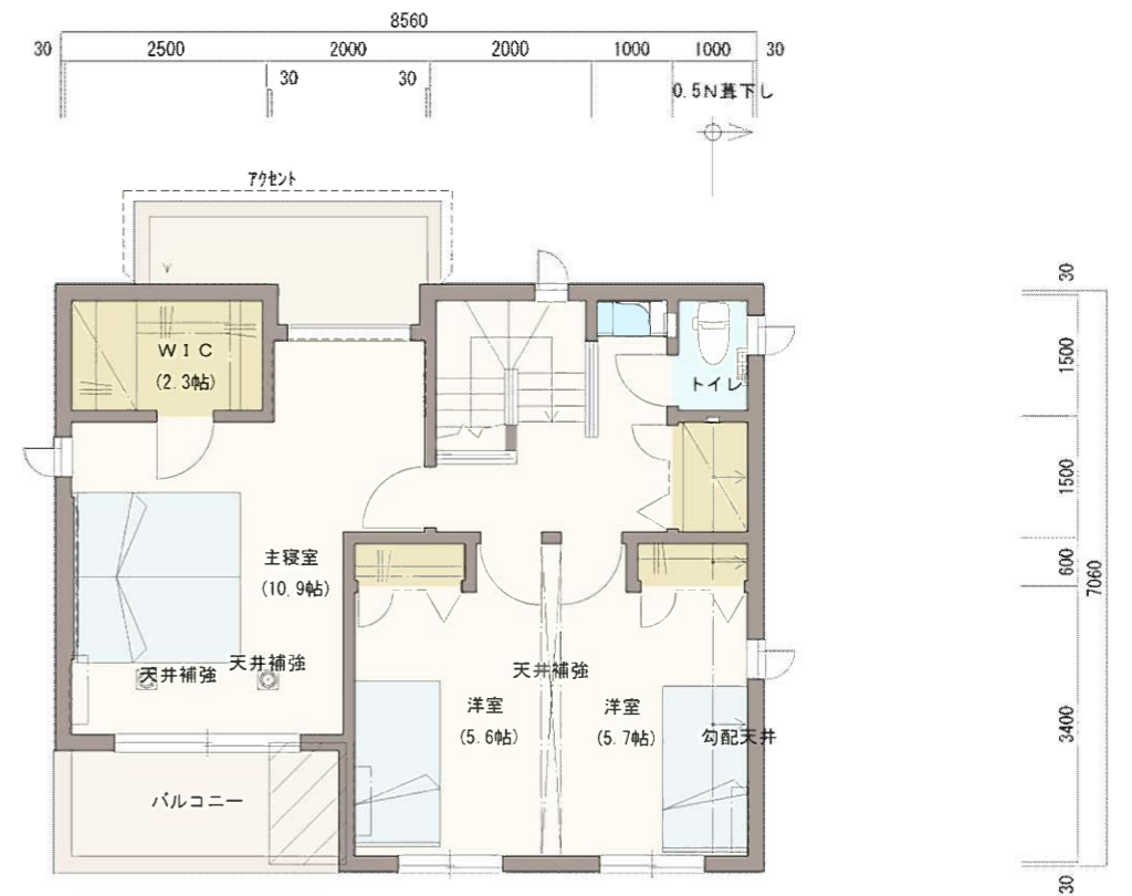
2階平面図 1/100
